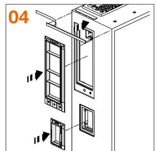
04 Einsetzen der Tunnelschieber AAR und RfZ (bei eHZ) sowie Ankleben der Verbindungsichtung (bei ZM01MS und ZM02MS inkl.)
