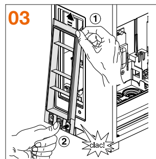
03 Einsetzen des Tunnelschiebers NAR
